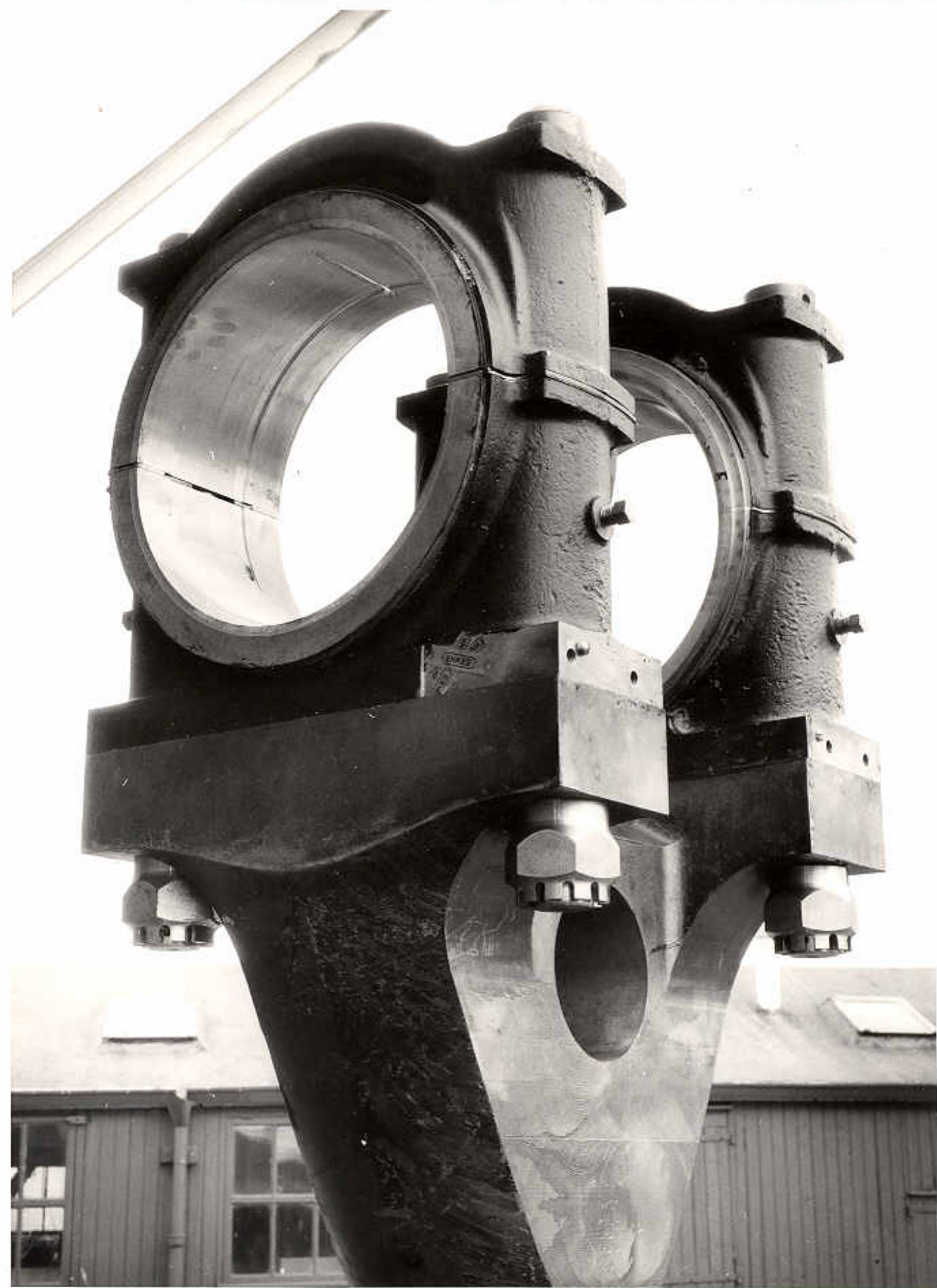
HET BEWERKEN VAN D M.A.N. DRIJSTANGEN
