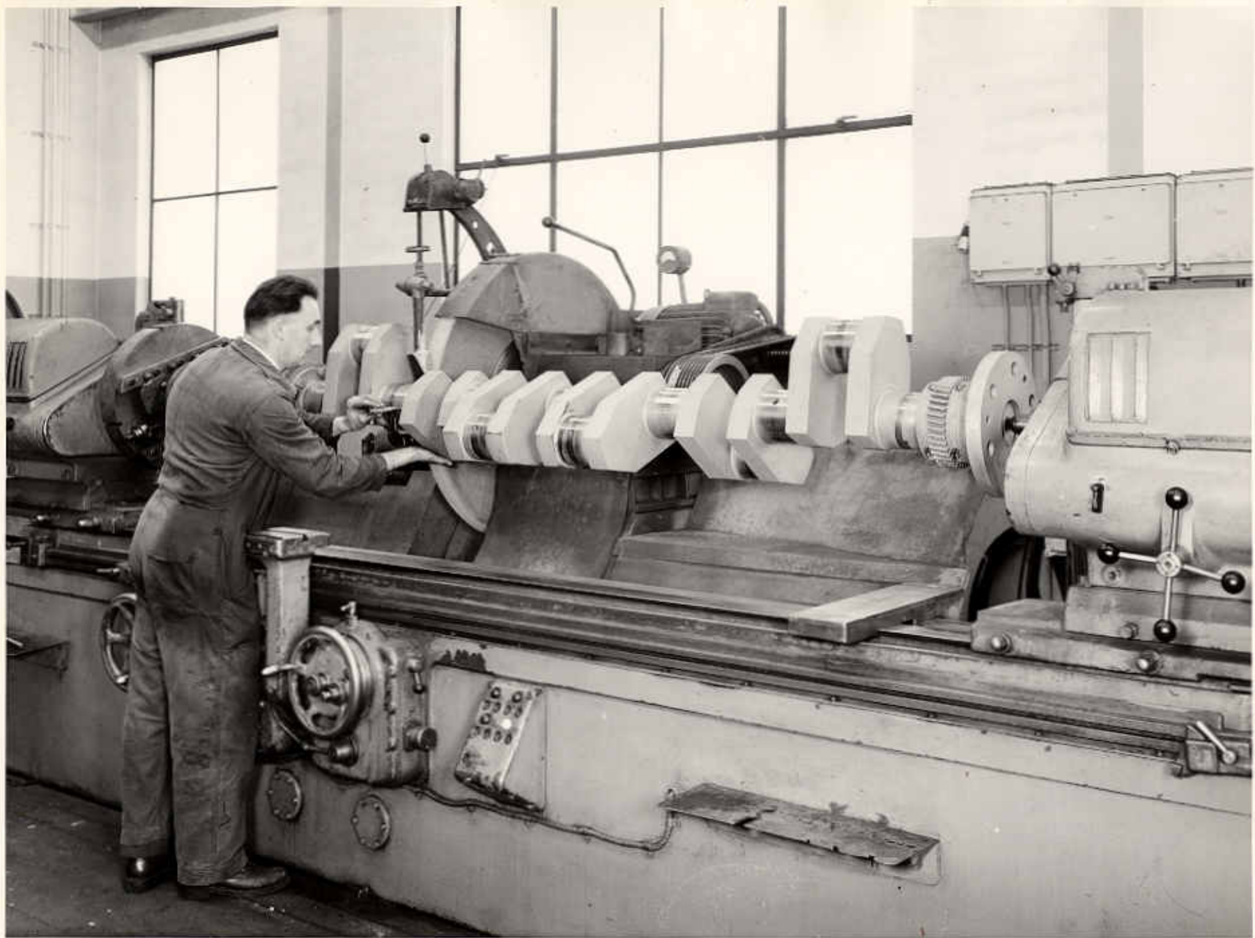
GEDEELTE VAN DE RUIM 9 METER LANGE KRUKASSEN-SLIPBANK
